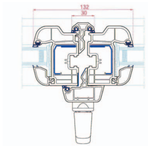
Sección Central
